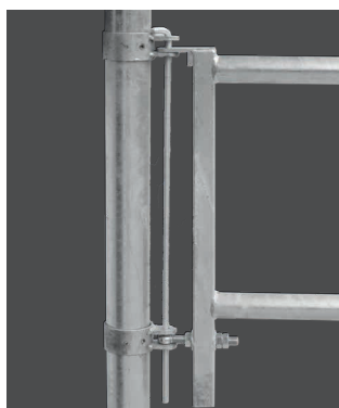
Standardeinschub
