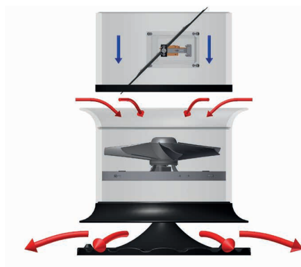
Stufe 2 Mischluft Produktionsphase
