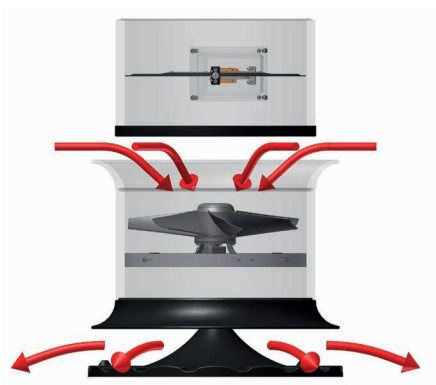
Stufe 1 Nur Umluft Aufheiz- und Startphase
